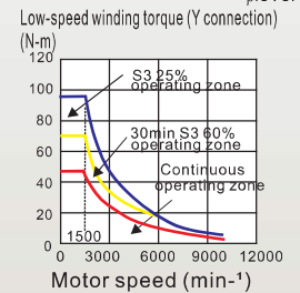
Spindle Motor
