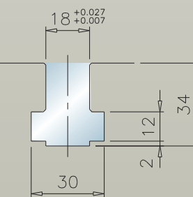
CV-2000 T-Slot dimensions
