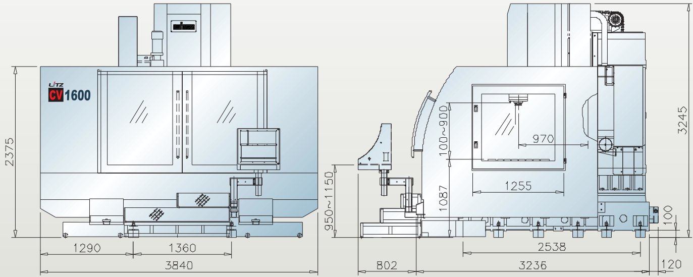
CV-1600
