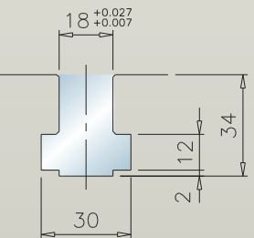
CV-1600 T-Slot dimensions
