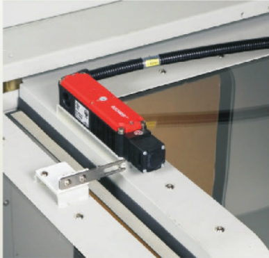
Safety Door Interlock
