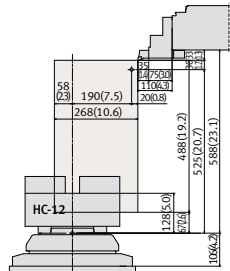
OD tool holder range
