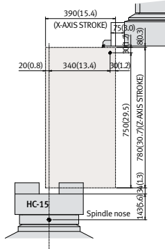
Extended OD tool holder range
